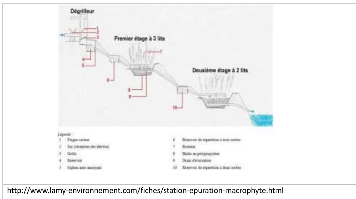
Figure 22: procédé de phytoépuration
