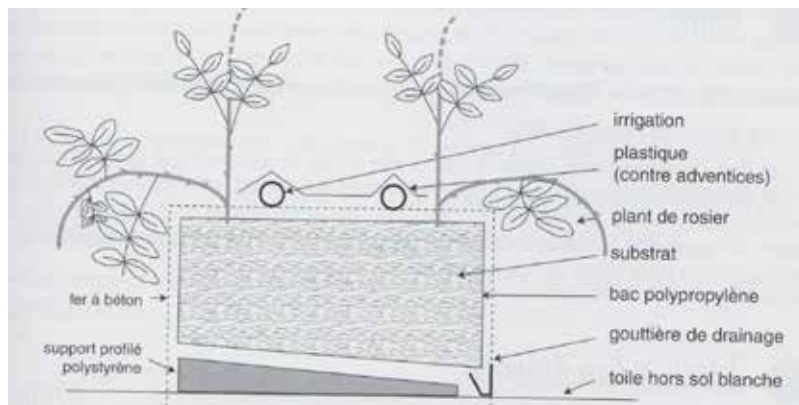
Coupe technique : culture de rose en Hors sol
