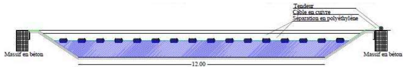
FIGURE 7. COUPE TRANSVERSALE DU BASSIN DE MATURATION
